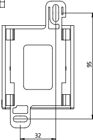
Vista posterior
